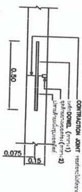
รอยต่อเพื่อการก่อสร้างหรือเพื่อการหดตัว (Construction Joint or Contraction Joint)
