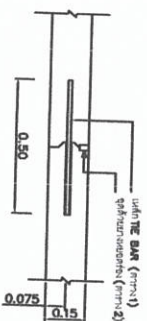
รอยต่อตามยาว (Longitudinal Joint)
