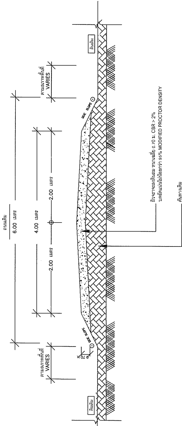
scale no scale รูปตัดแสดงโครงสร้างถนนดินถม
