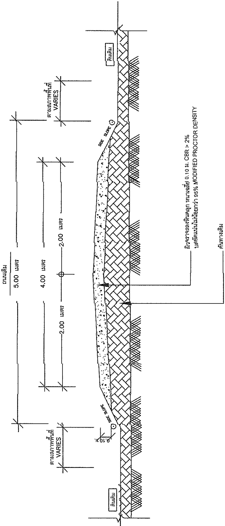
รูปตัด แสดงโครงสร้างถนนหินคลุก
